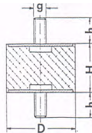
Puffer, zylindrisch Typ B
