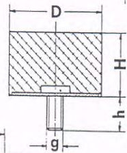
Puffer, zylindrisch Typ D
