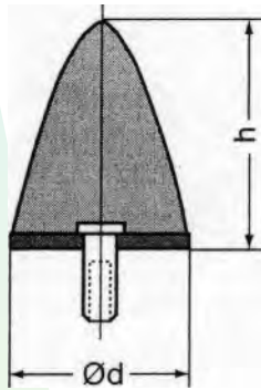
Gummi-Metall-Puffer Ausführung „P“ (parabel)
