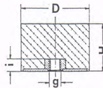
Puffer, zylindrisch Typ D
