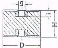
Puffer, zylindrisch Typ C
