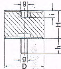
Puffer, zylindrisch Typ B
